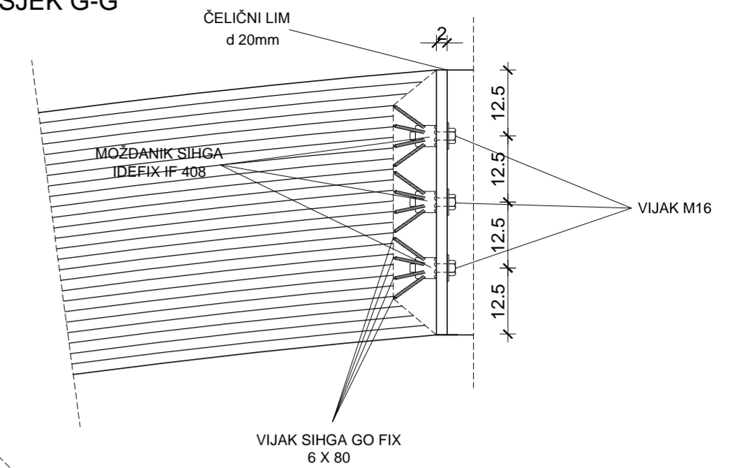
PRESJEK G-G
