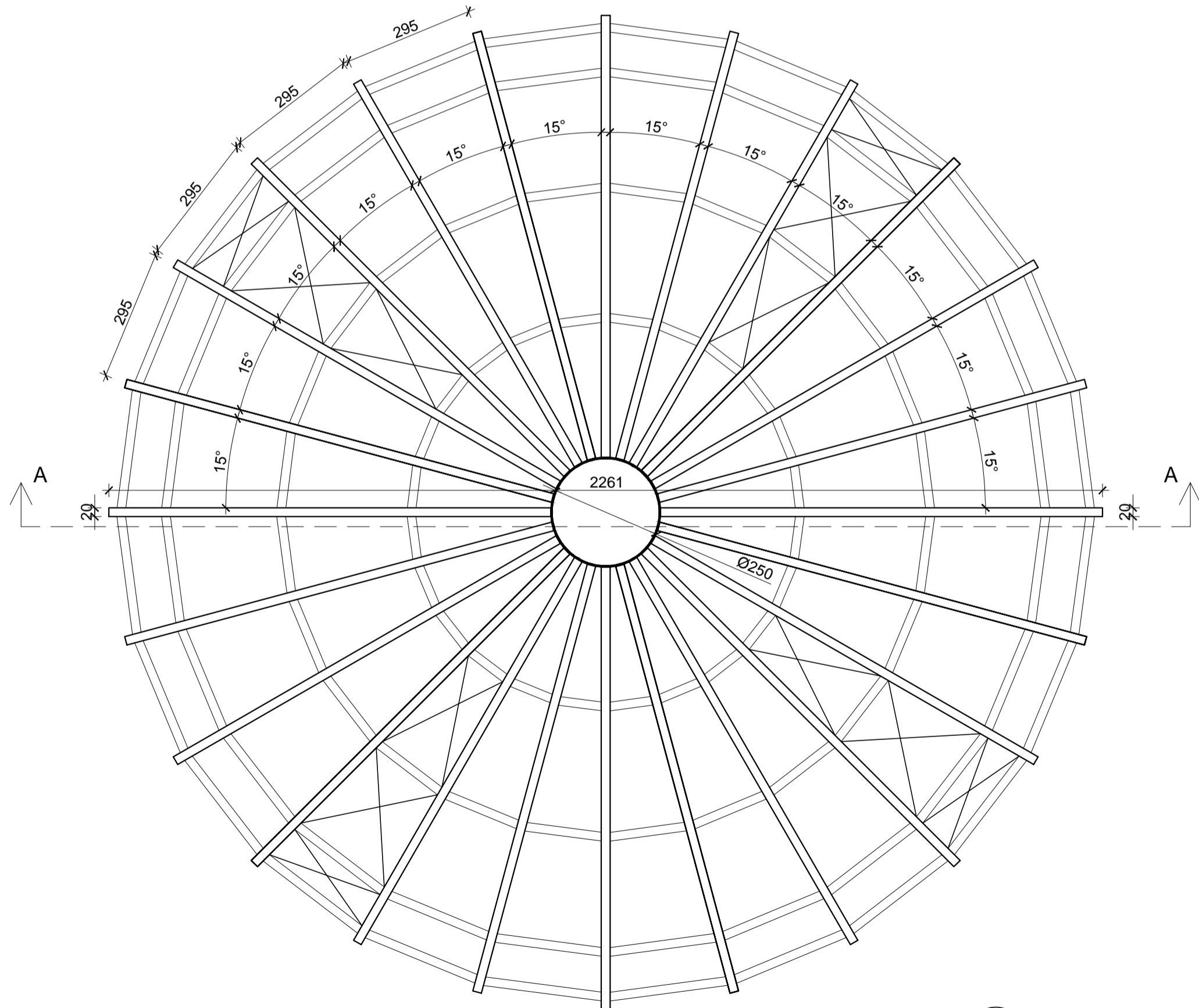
TLOCRTNA DISPOZICIJA
